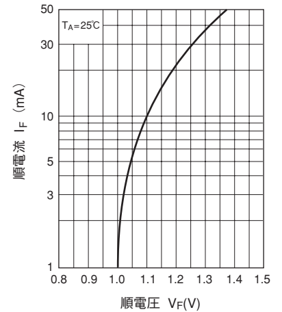
順電流—順電圧特性 (標準値)
