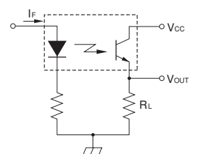
※応答時間測定回路 Switching Time Test Circuit
