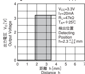
検出位置特性 (1) (参考)
