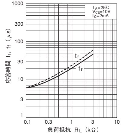
応答時間—負荷抵抗特性 (標準値)※3 Switching Characteristics (Typ.)
