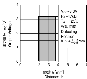
検出位置特性(1) (参考)
