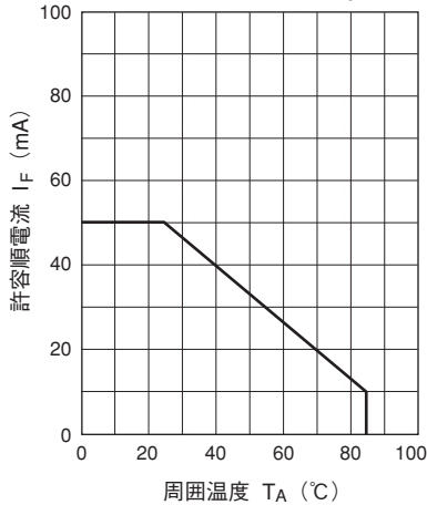
順電流低減曲線
