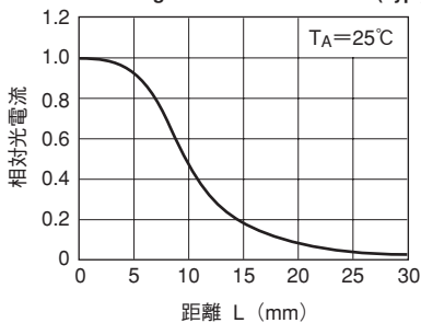
相対光電流—距離特性 (標準値) ※4 Relative Light Current vs. Distance (Typ.)
