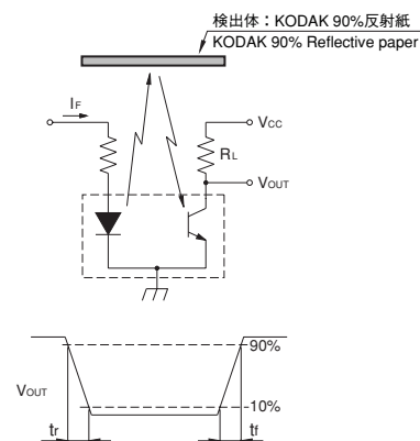
※4 応答時間測定回路 Switching Time Test Circuit
