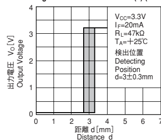
検出位置特性 (2) (参考)
