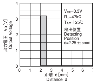
検出位置特性 (2) (参考)
