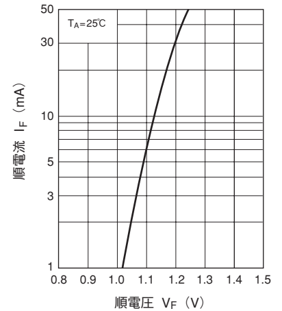
順電流—順電圧特性（標準値）
