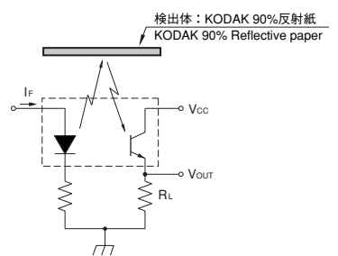
※4 応答時間測定回路 Switching Time Test Circuit
