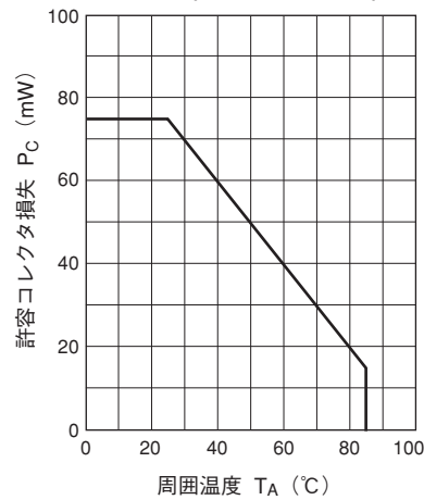
コレクタ損失低減曲線
