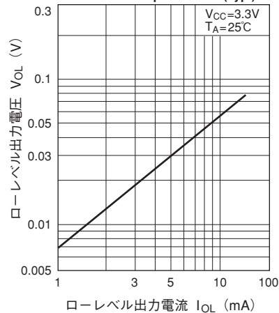
ローレベル出力電圧—ローレベル出力電流特性 (標準値)
