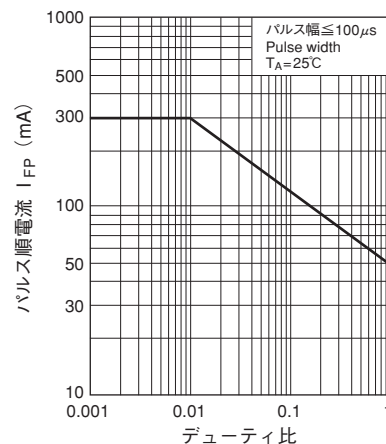
パルス順電流—デューティ比 Pulse forward current vs. Duty Ratio
