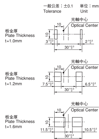
取り付け穴寸法 (参考) Installation Hole Dimensions (Reference)
