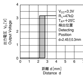
検出位置特性(2) (参考)
