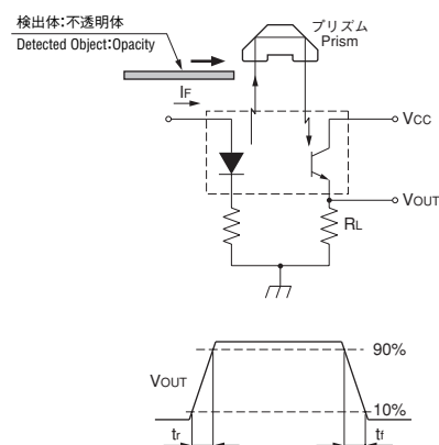
※3 応答時間測定回路 Switching Time Test Circuit
